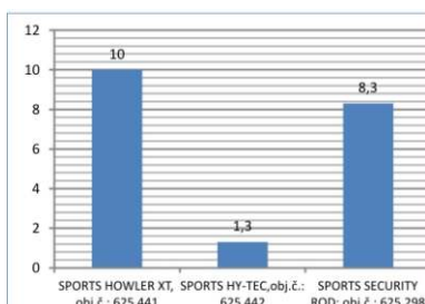
Citlivosť nastavená na MIN rozpoznanie záberu v cm
