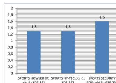
Citlivosť nastavená na MAX rozpoznanie záberu v cm
